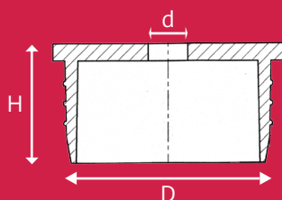
Réducteur de débit Flow plugs
