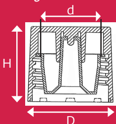
Bouchon distributeur Stiligoutte Dispensing closure Stiligoutte
